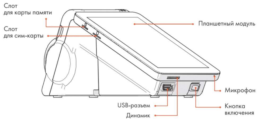
Смарт-терминал «Эвотор 7.2», вид спереди и сбоку
